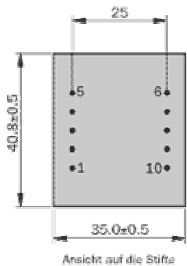
Ausführung „0“ Vergußgehäuse ohne Befestigungslaschen
